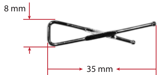
METAL CLIPS-NO:2/C
